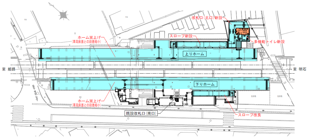
<中八木駅 平面図>
