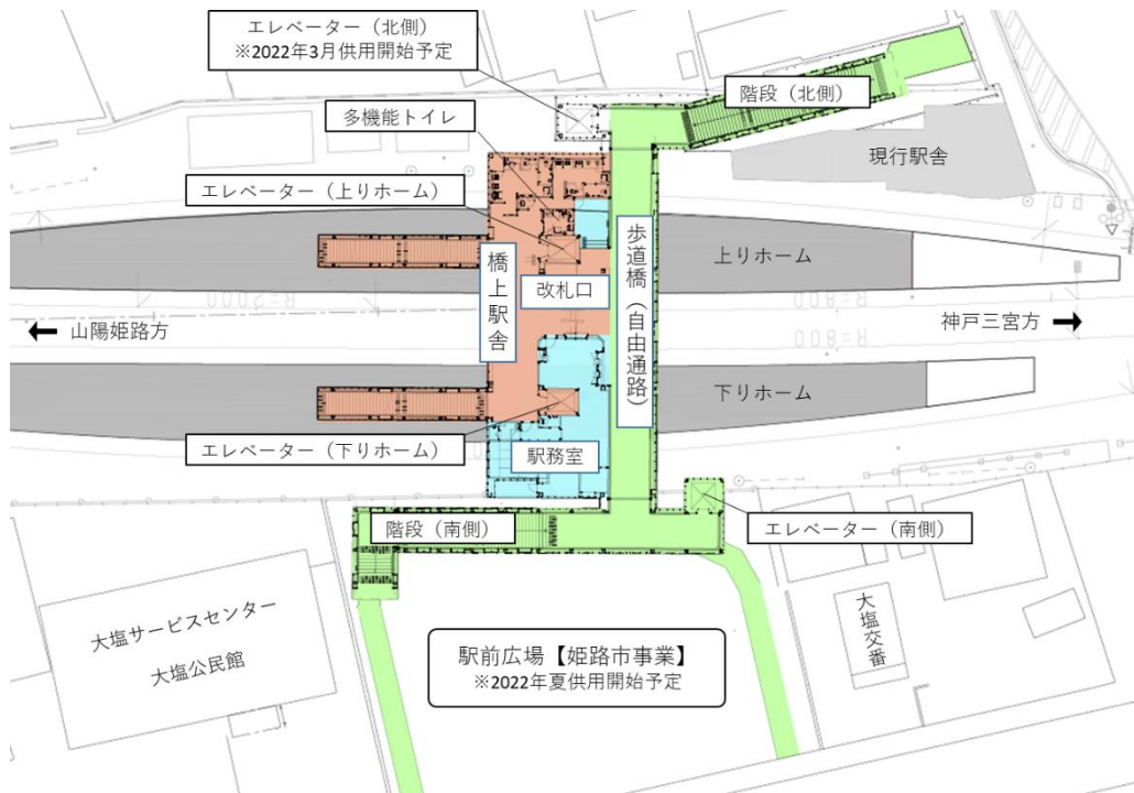
橋上駅舎・歩道橋 平面図
