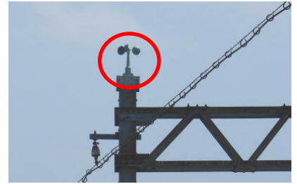
橋りょう上に設置している風速計
