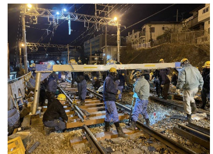
山陽須磨駅12号分岐器更新工事
