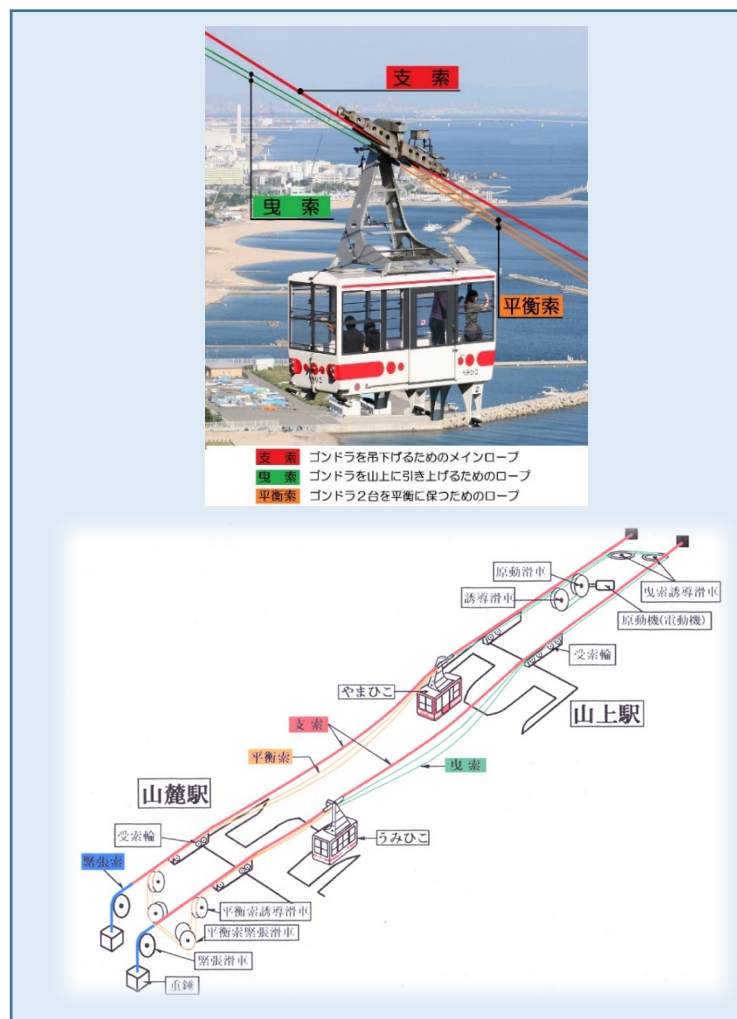
ロープウェイの仕組み
