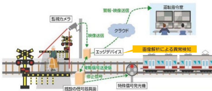
A I 画像解析を用いた人特化型踏切障害物検知システム
