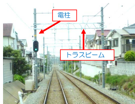
更新された藤江駅～中八木駅間の支持物
