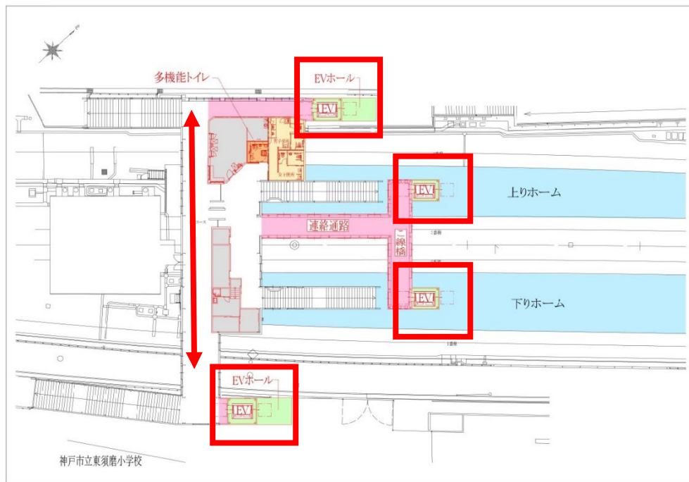
東須磨駅 平面図
